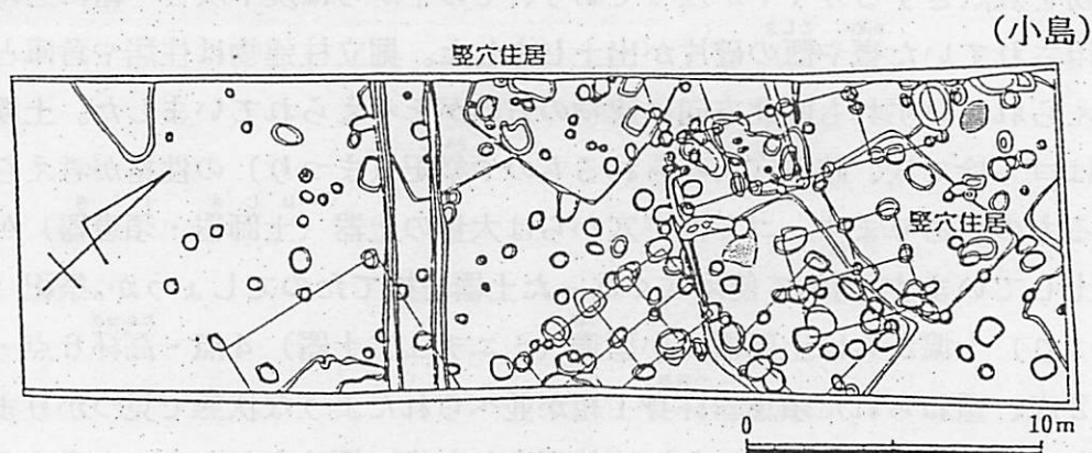
阿比留遺跡西側調査区遺構平面図
