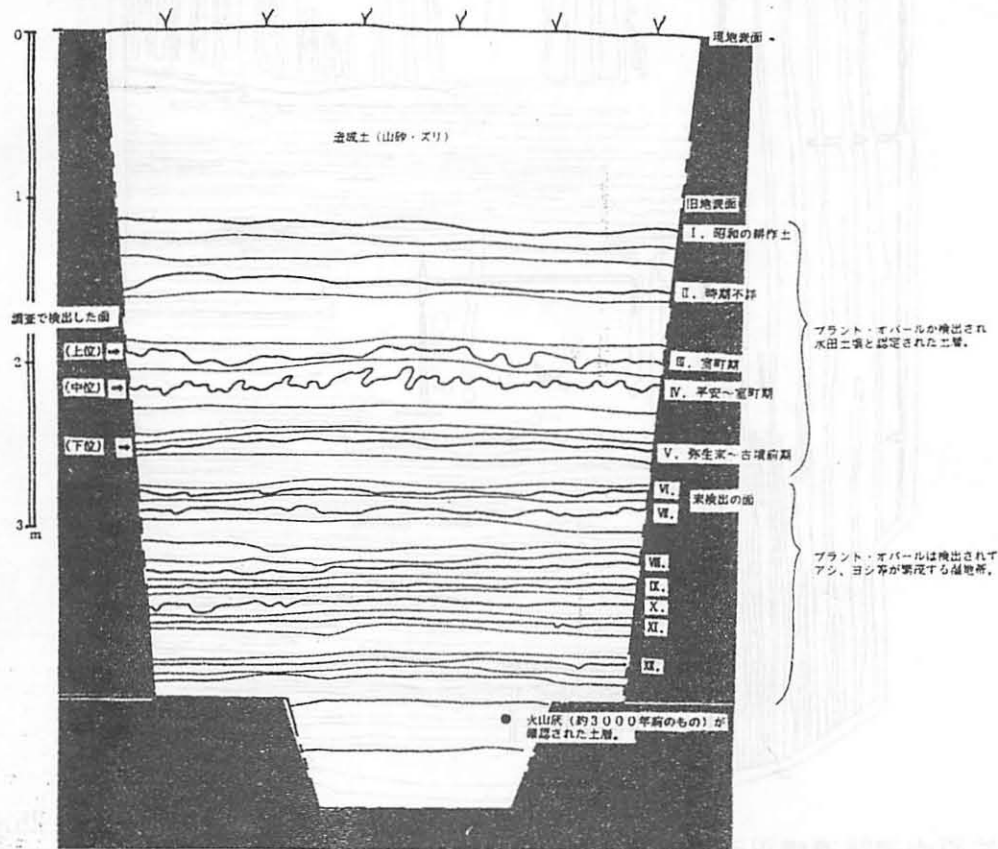
笠原南遺跡土層断面図
